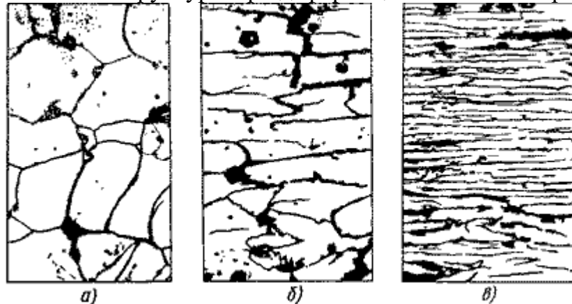
Рис. 8.1. Изменение структуры при деформации: а) до деформации; б) после обжатия на 35%; в) после обжатия на 90%.
